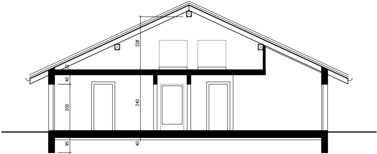
COUPE A-A
